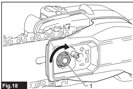
Fig.18 1. Écrou de retenue
