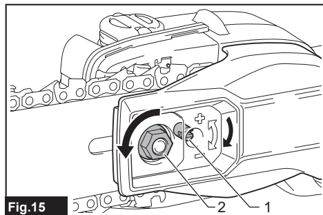
Fig.15 1. Vis de réglage de la chaîne 2. Écrou de retenue
