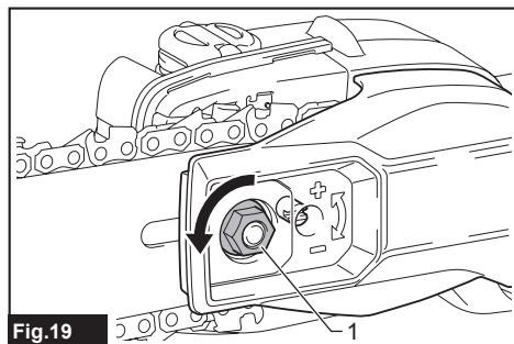
Fig.19 ► 1. Tuerca de retención
